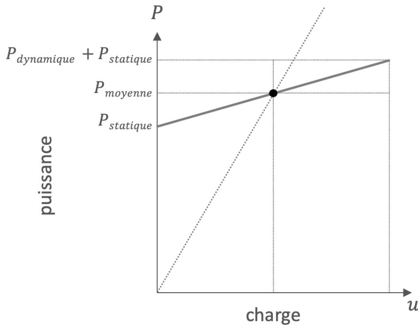
Puissance électrique typique d'un serveur de calcul en fonction de sa charge processeur (tracé gris).
